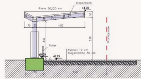
Schnitt B-B 1:100
