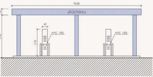
Ansicht Stromtankstelle 1:100
