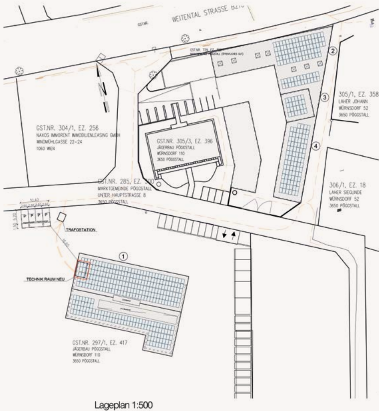
Lageplan 1:500
